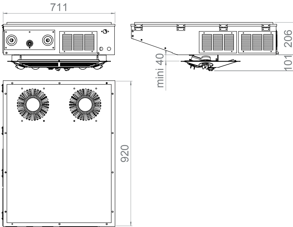
Plafonier / Ceiling panel
